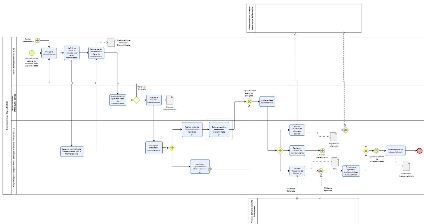
Figura 1 – Fluxo do Processo de Gerenciamento de Disponibilidade
