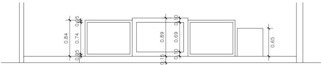
Vista Frontal – Bancada Sem escala
