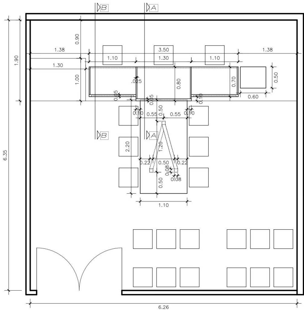
SALA DE AUDIÊNCIA 01 – Planta Layout Sem escala
