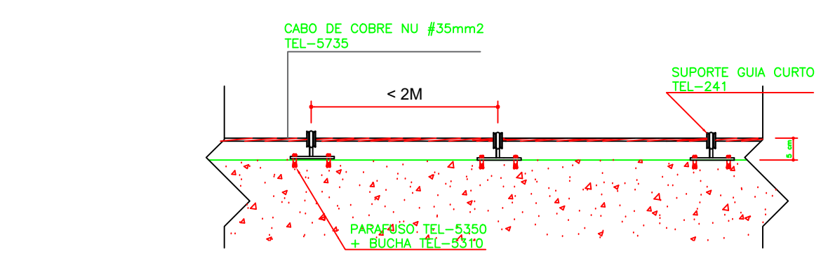
DETALHE F: CABO FIXADO ATRAVÉS DE SUPORTE GUIA CURTO SEM ESCALA
