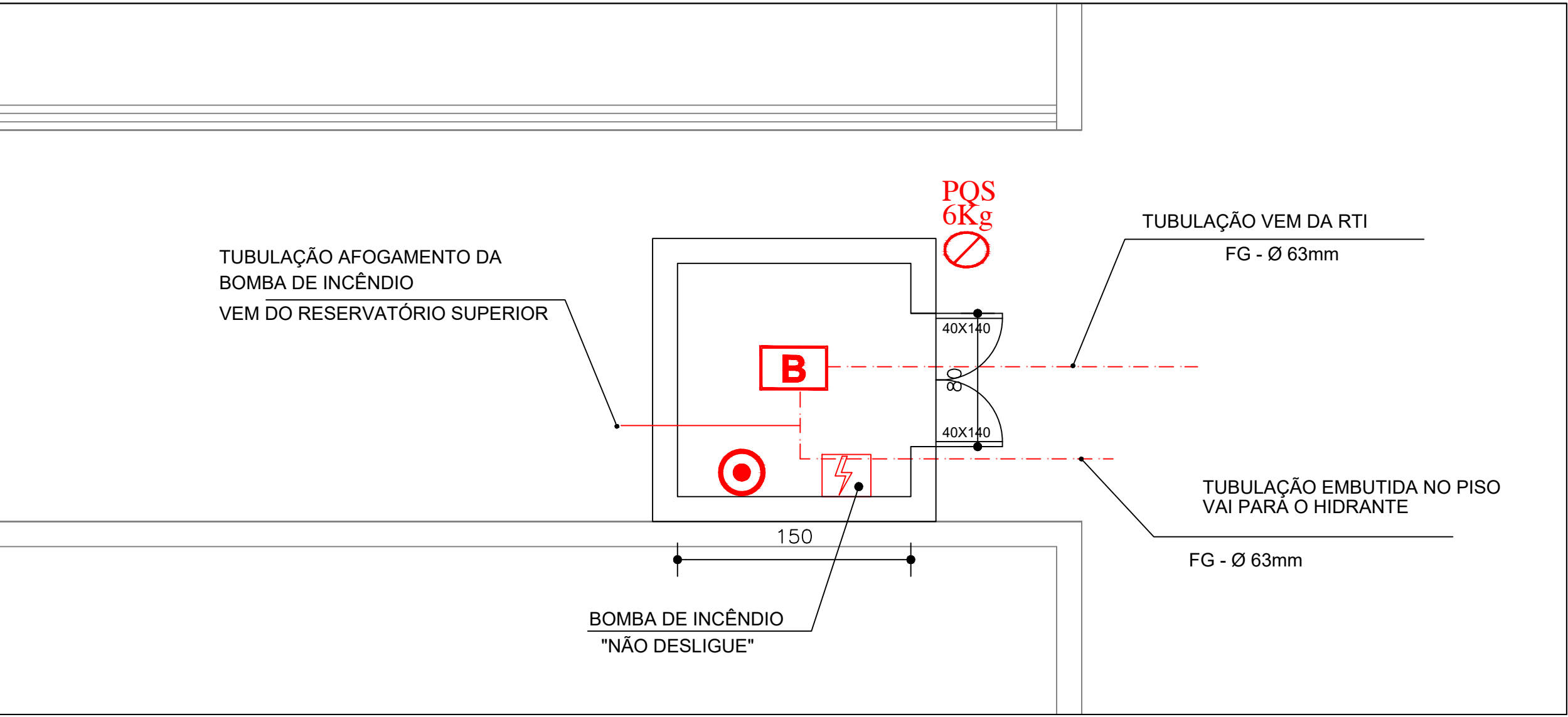
CASA DE BOMBAS SEM ESCALA
