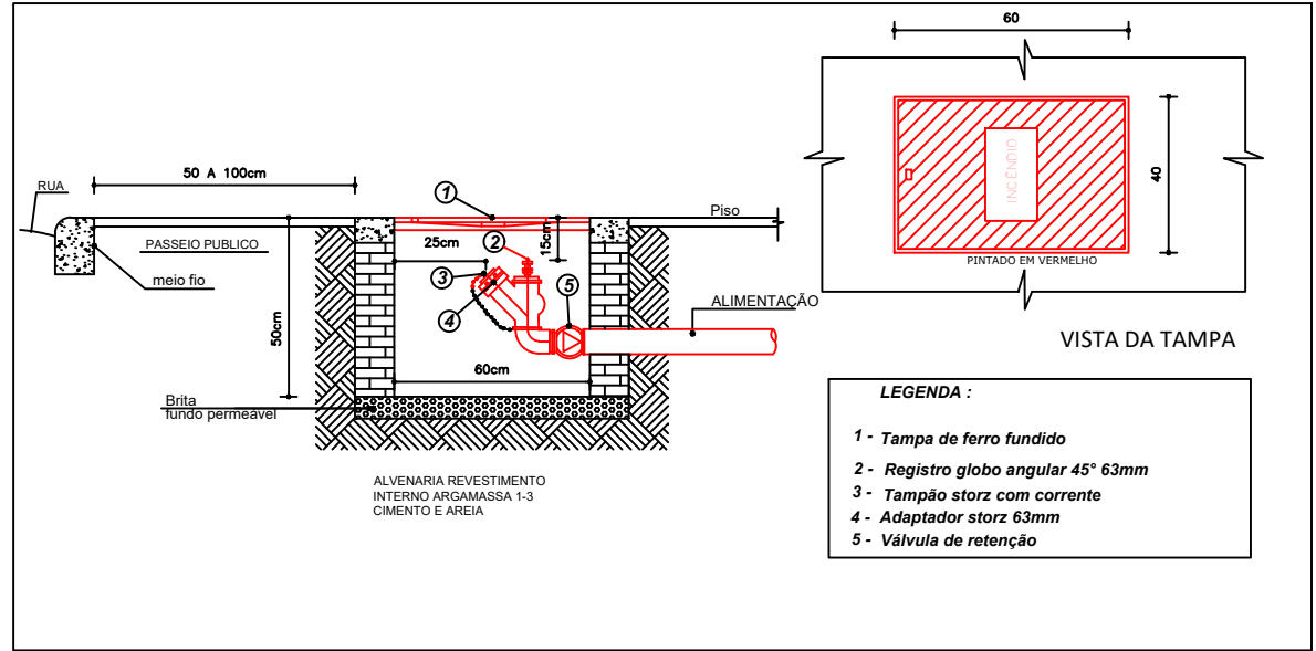
DET. HIDRANTE DE RECALQUE SEM ESCALA
