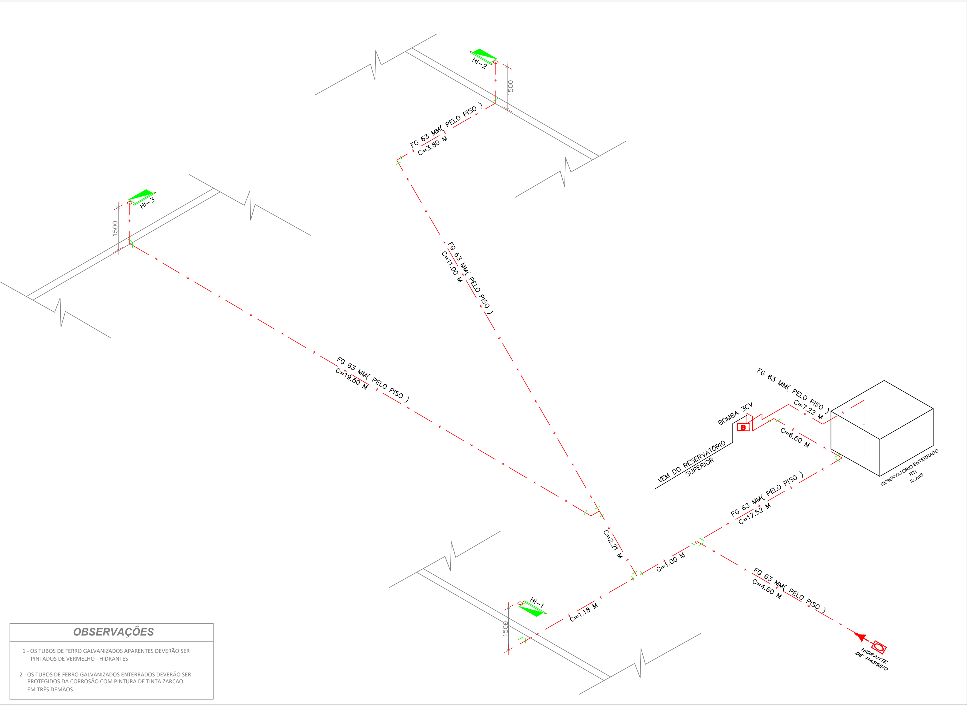
DETALHE GENÉRICO ISOMETRIA DAS LIGAÇÕES DOS HIDRANTES SEM ESCALA
