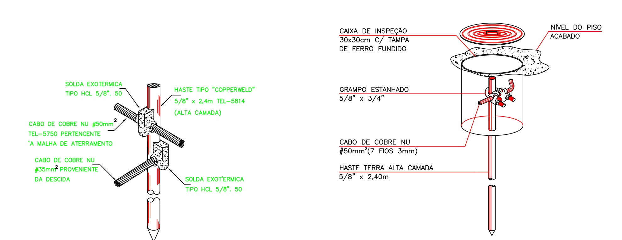
DETALHE H: CAIXA DE INSPEÇÃO SEM ESCALA
