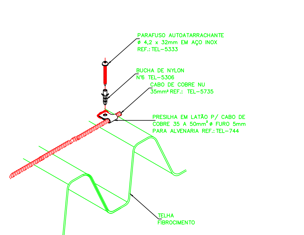
DETALHE G: CABO DE COBRE NU EM TELHA DE FIBROCIMENTO SEM ESCALA
