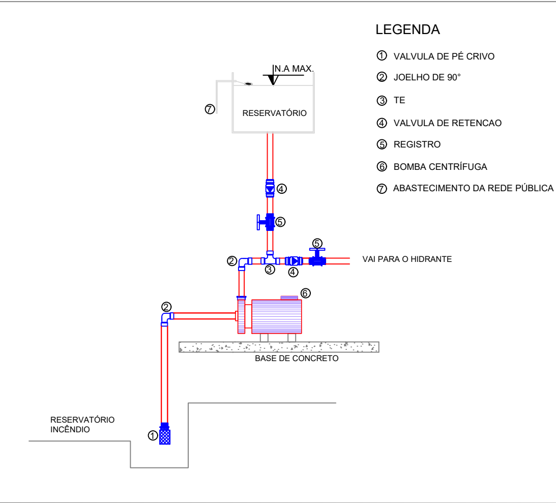
ESQUEMA AFOGAMENTO DE BOMBA DE INCÊNDIO Sem escala
