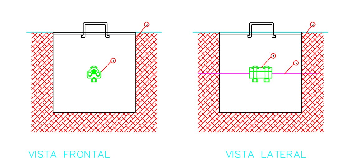
DETALHE D: CAIXA DE INSPEÇÃO DE TERRA SEM ESCALA
