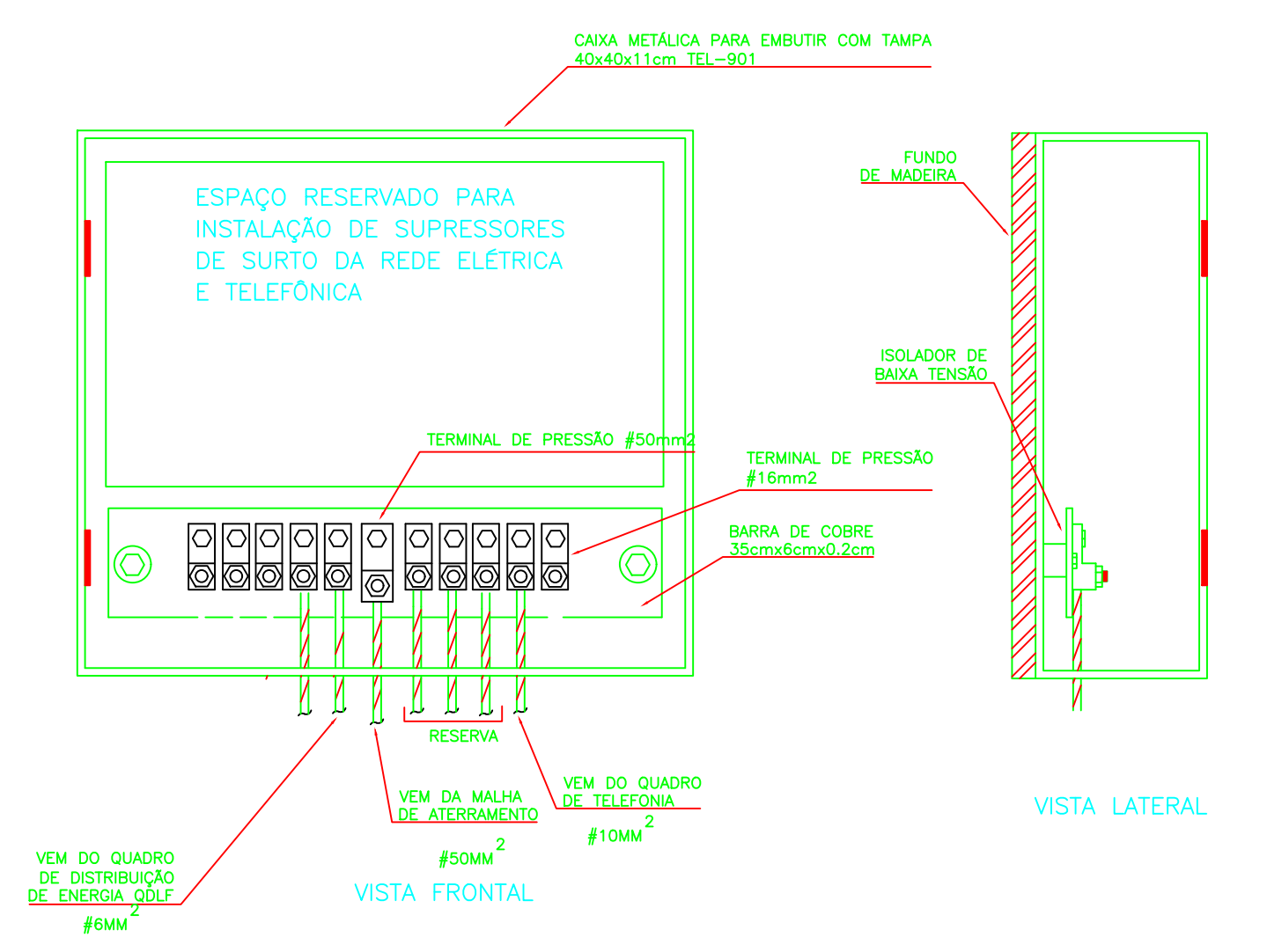
DETALHE B: CAIXA DE EQUALIZAÇÃO SEM ESCALA
