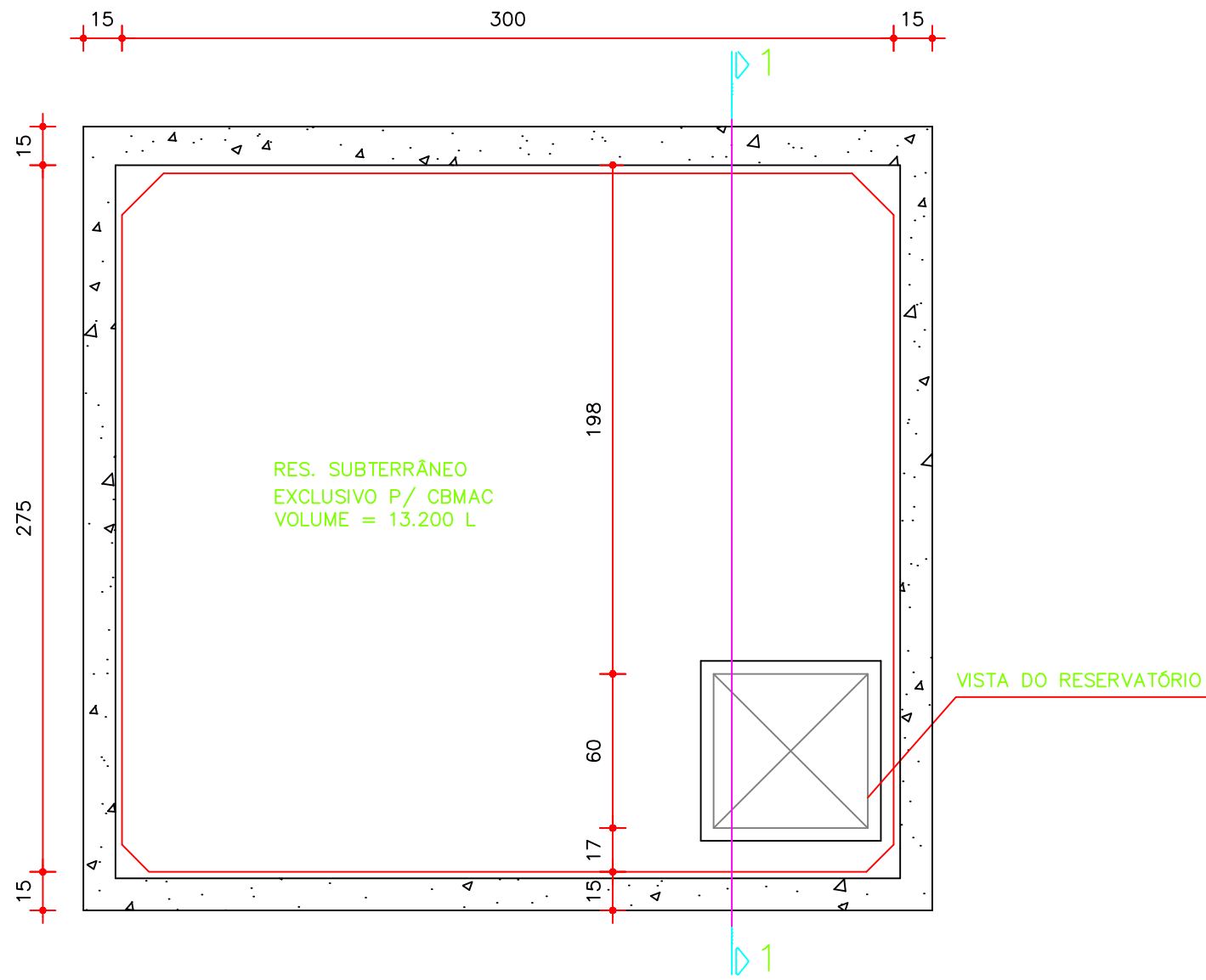
PLANTA BAIXA-RESERVATÓRIO DE INCENDIO CAPACIDADE: 13.200 LITROS ESCALA 1:25
