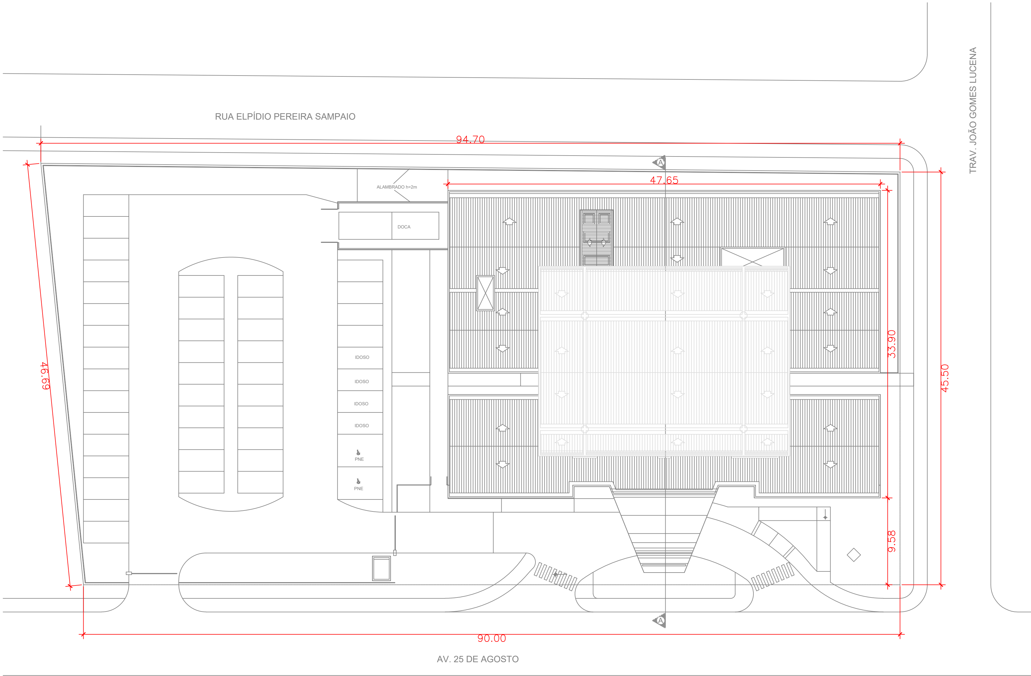
PLANTA COBERTURA E LOCAÇÃO ESCALA 1:250
